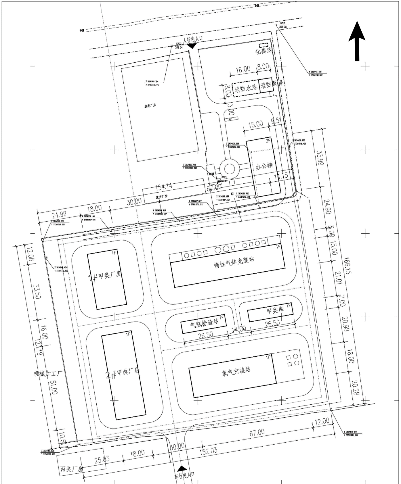
附图3 总平面布置图
