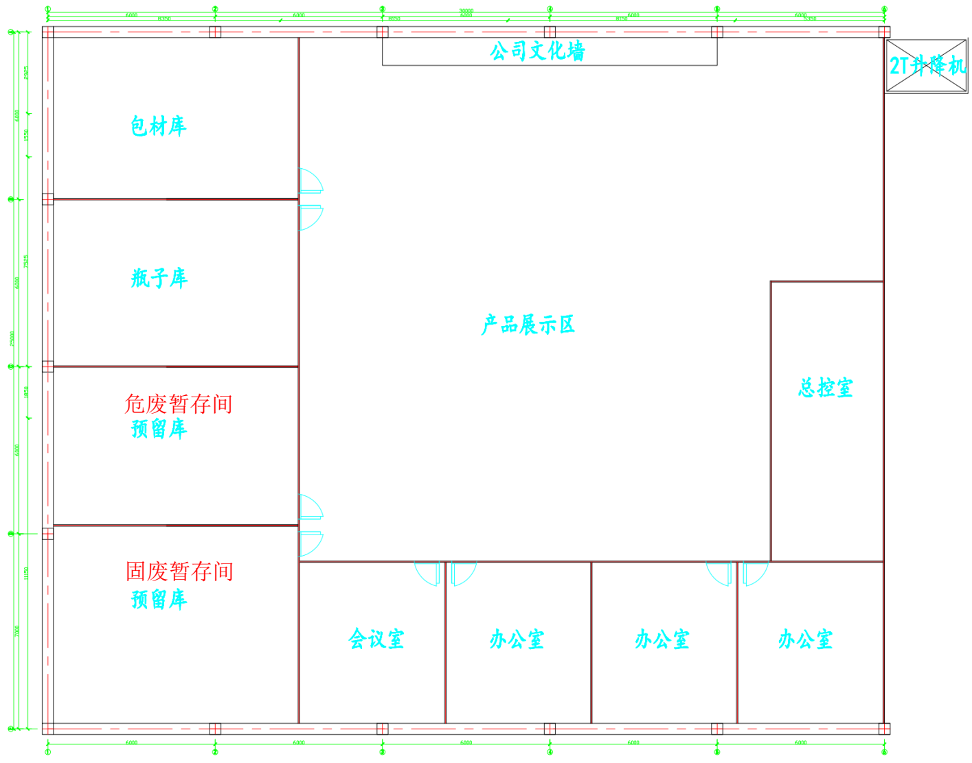
附图 4-2 项目总平面布置图 (二层)
