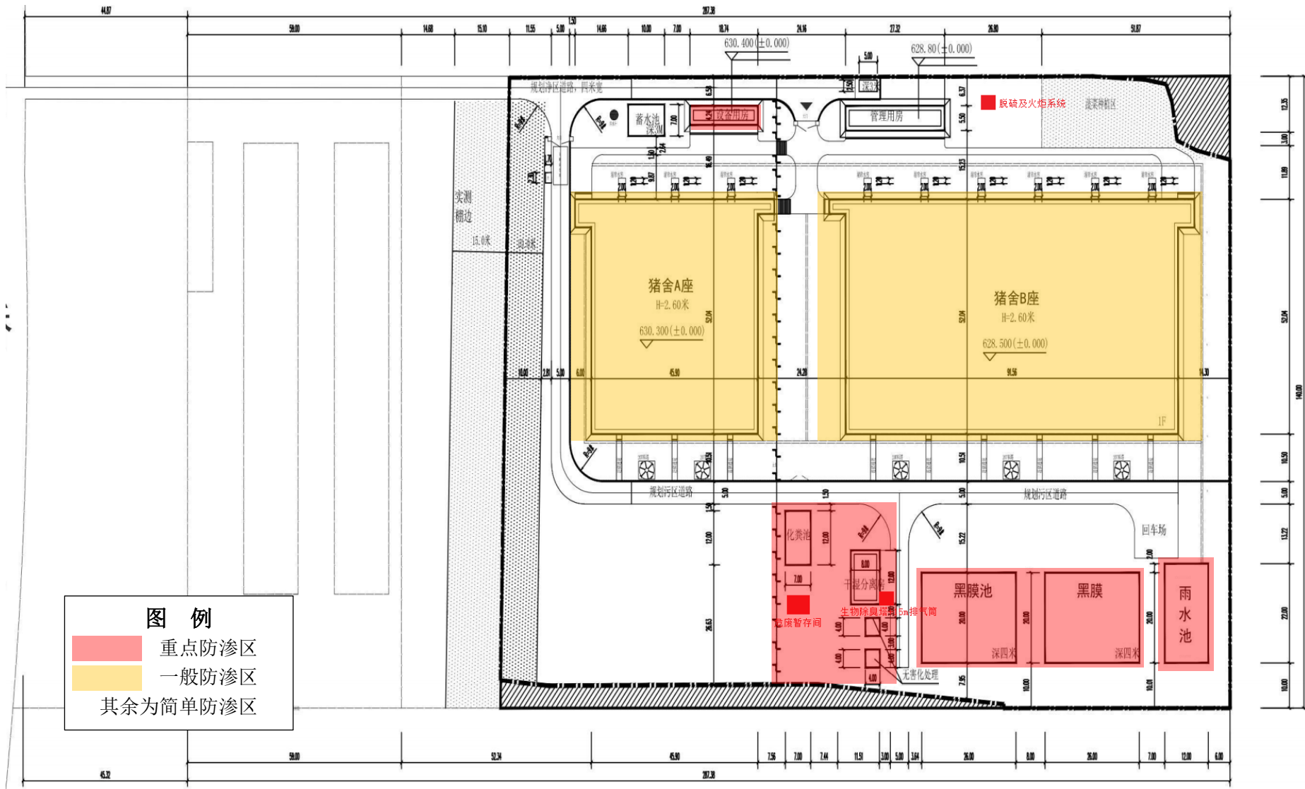
附图 7 项目分区防渗图
