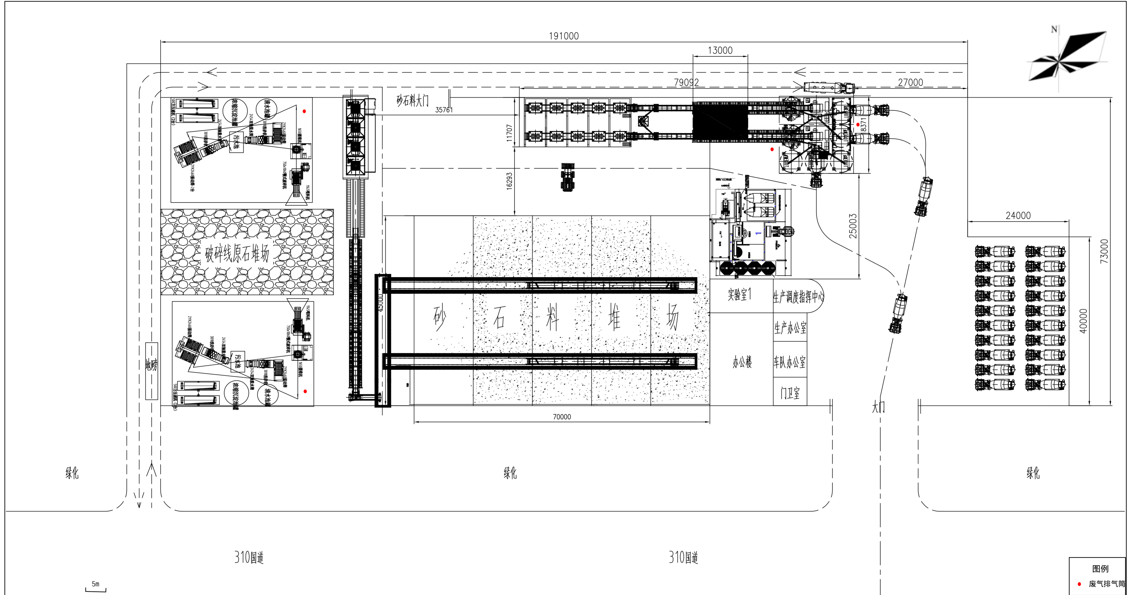
附图3-1 项目(1#生产区)平面布置示意图
