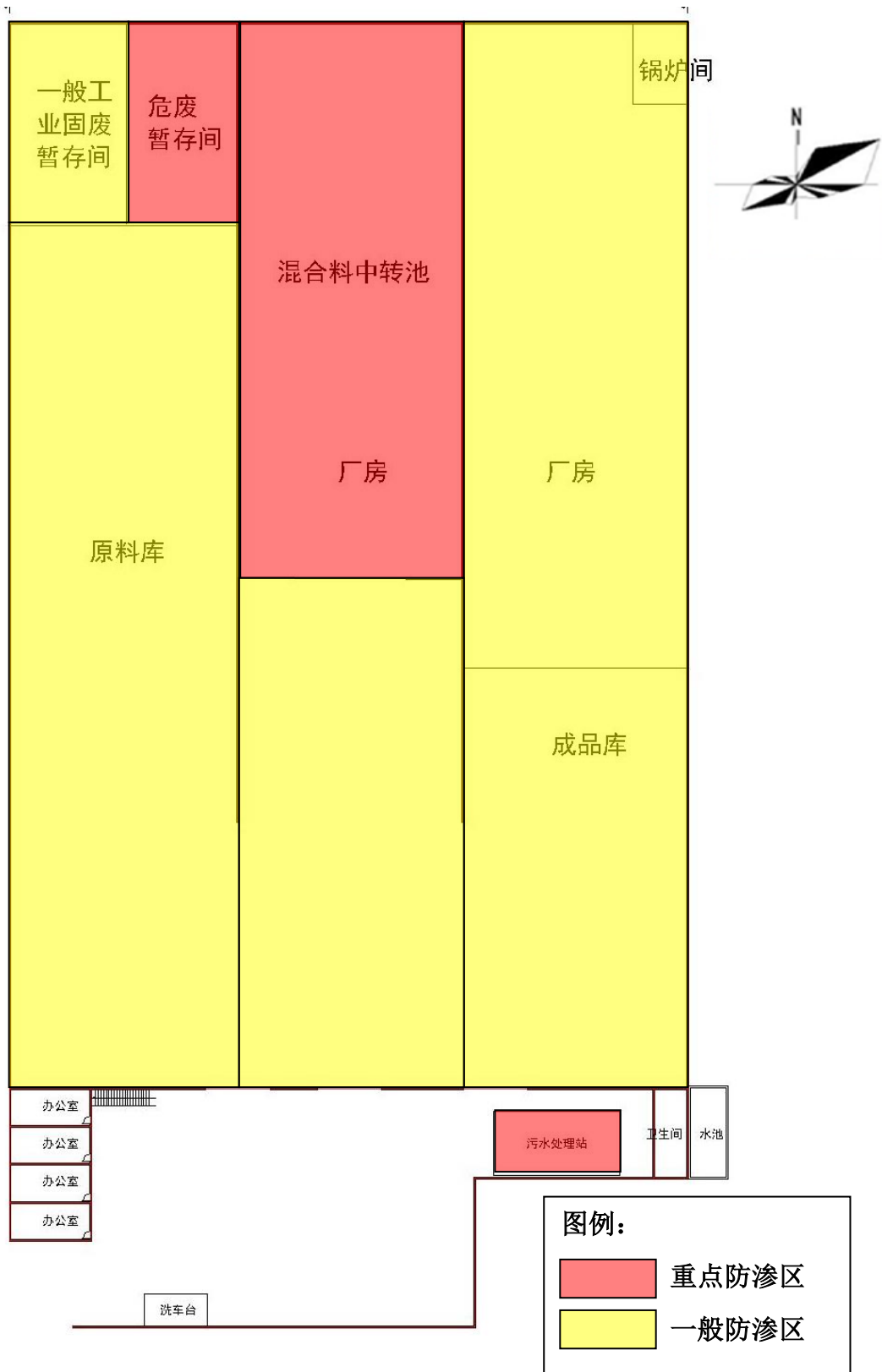
附图 6 分区防渗图
