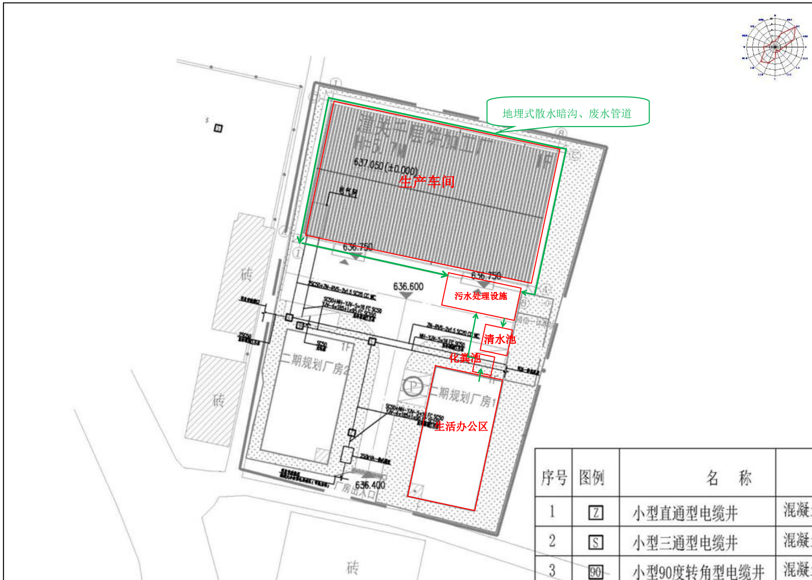
附图 4-1 项目平面布置图 (一)
